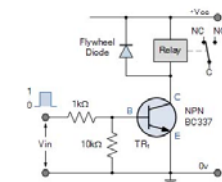
Saklar Elektronik Sederhana Menggunakan Relay
