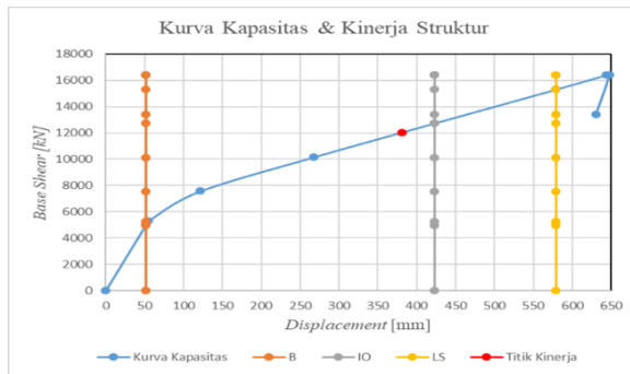
Gambar 5. Kurva Kapasitas dan Kinerja Struktur Cast in Situ tanpa Base Isolator Arah UX
