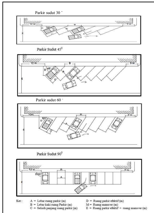
Gambar 3. Parkir membentuk sudut 30^\circ , 45^\circ , 60^\circ , dan 90^\circ (Sumber: Direktorat Jenderal Perhubungan Darat, 1998)
