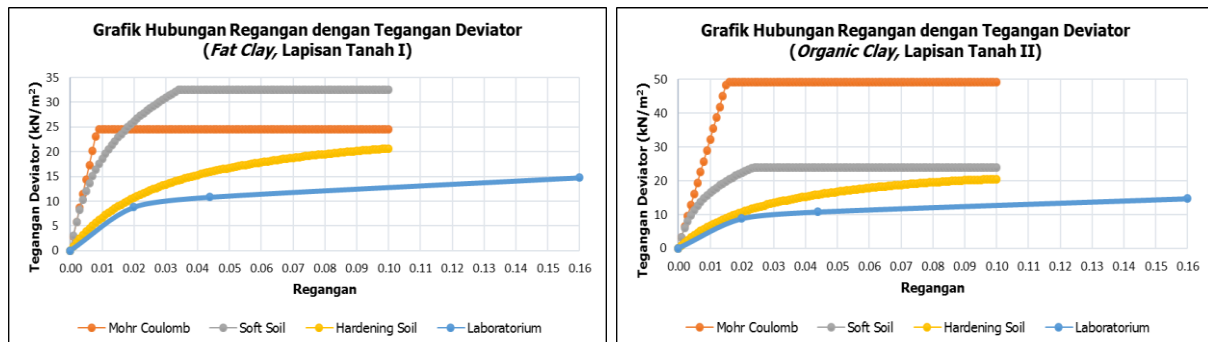
Gambar 10. Grafik hubungan regangan dengan tegangan deviator
