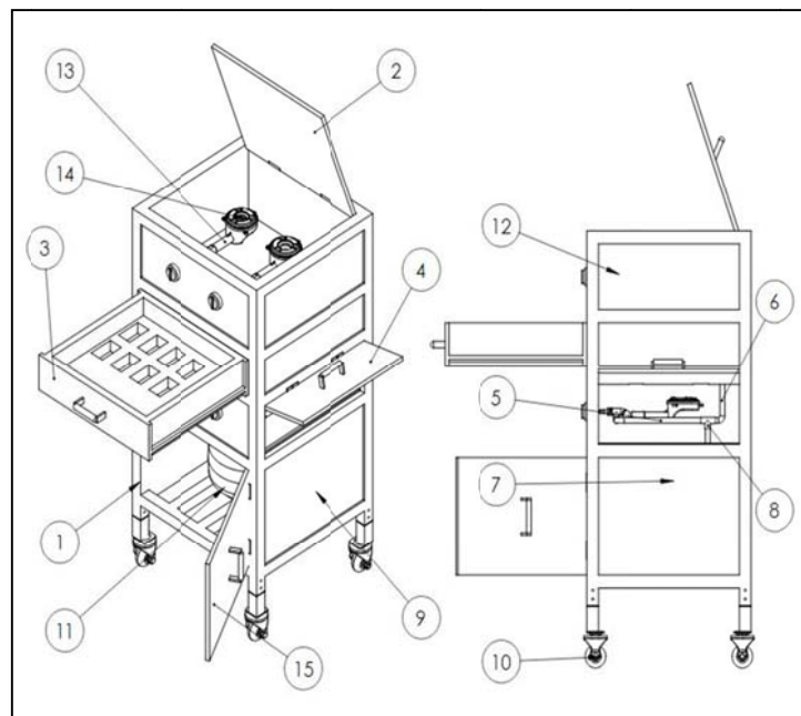
Gambar 11. Alat Panggang Kue Balok Rancangan 3
