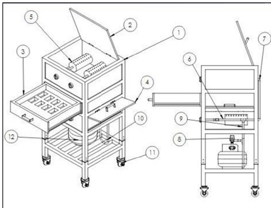
Gambar 3. Alat Panggang Kue Balok Rancangan 1
