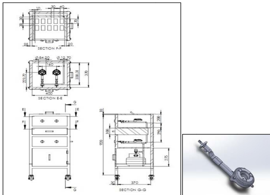
Gambar 14. Alat Panggang Kue Balok Rancangan 3 dan Tungku Bulat.
