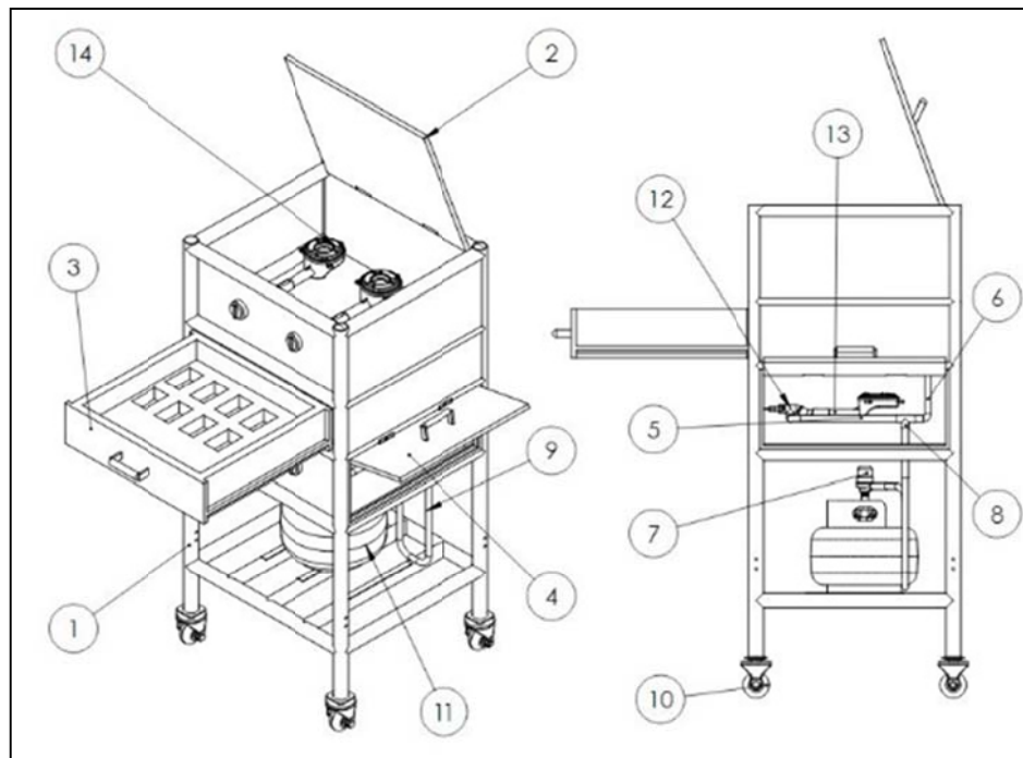
Gambar 7. Alat Panggang Kue Balok Rancangan 2
